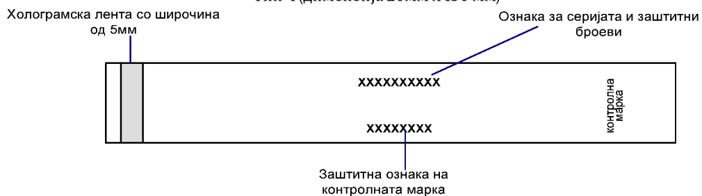
Тип 4 (димензија 20мм x 130 мм)
